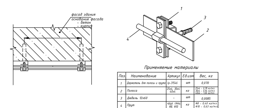
Узел фиксации токоотвода. Конструкция дает возможность крепить как прут так и полосу
