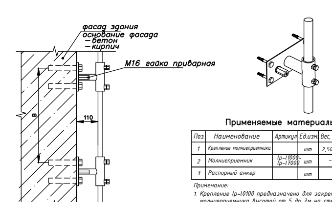
Узел крепления молниеприемника к стене
