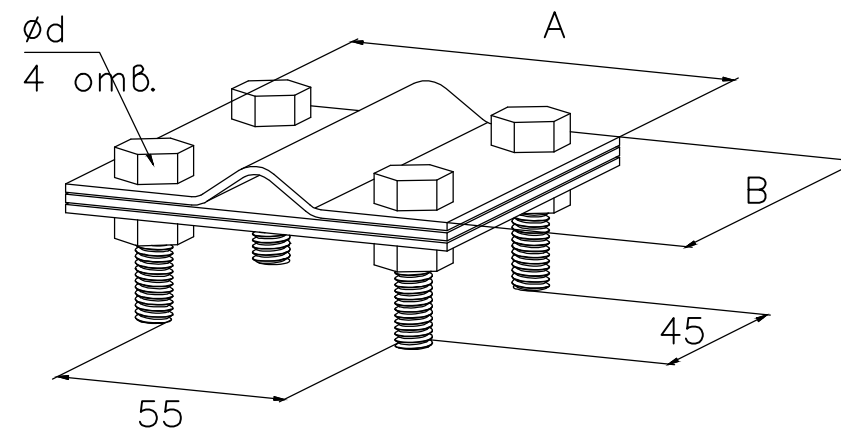
Зажим "заземлитель 20 - полоса 50"
