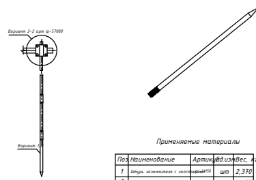
Узел крепления штыря заземлителя с заострением
