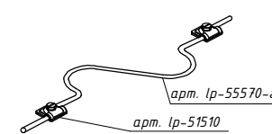
Установка компенсаторов теплового расширения каждые 20 м на прямолинейных участках
